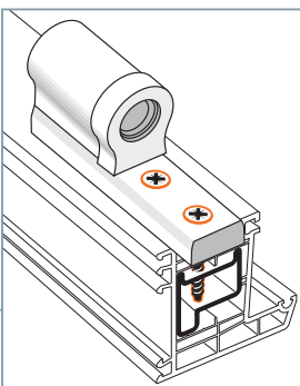
Scharnierdeel op het deurka- der schroeven.
