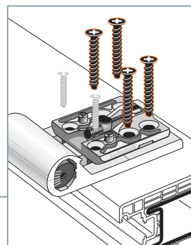
Scharnierdeel op de deur vast Schroeven.
