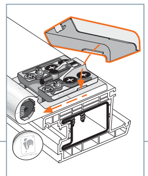
Afdeksluk plaatsen.
