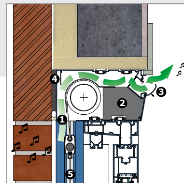
DOORSNEDEN
