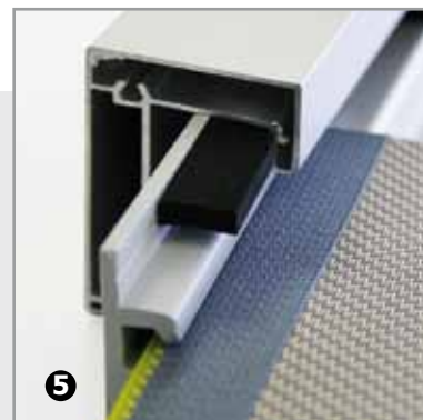
DETAIL GELEIDINGSSYSTEEM
