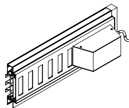
Motorbediening Breedte: 152 mm Hoogte: 63 mm Diepte: 62 mm
