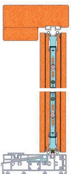
Technische omschrijving schuif- en ontgrendelings- positie.
