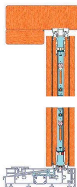
Gesloten stand sluitelementen vergrendelen aan boven en onderrail.
